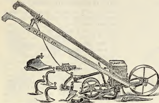
No. 4.—Planet, Jr.
